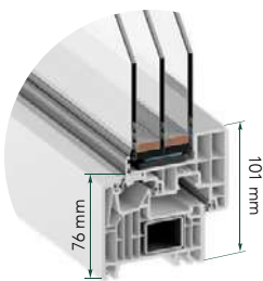
Nodo laterale
