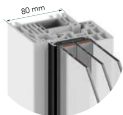
Nodo laterale
